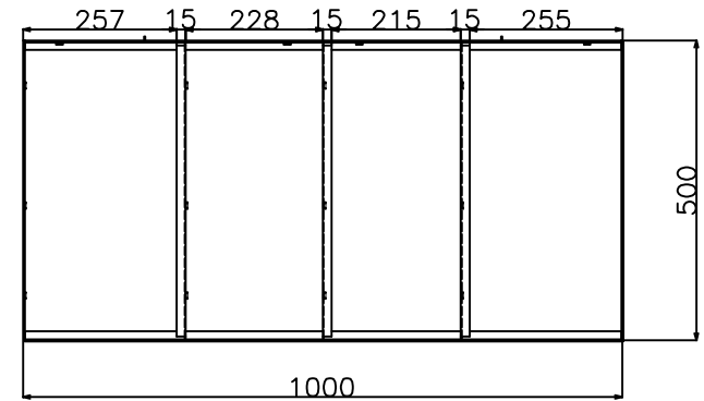
背面図
