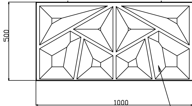
正面図
