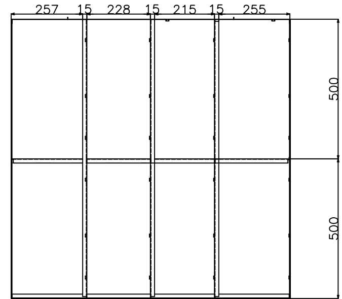
鋼製有孔型枠 (ブラインド加工鋼板) 詳細図
