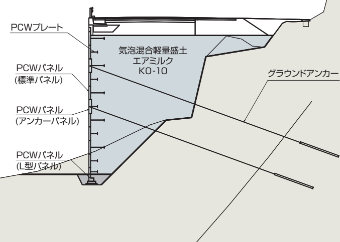
標準断面図
