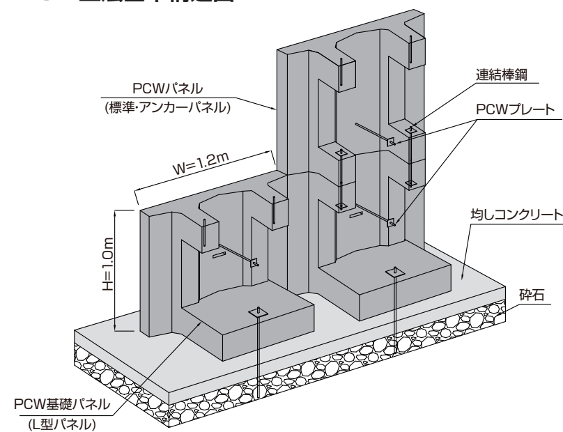
PCW工法基本構造図
