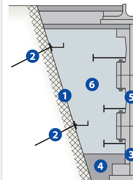
標準断面図
