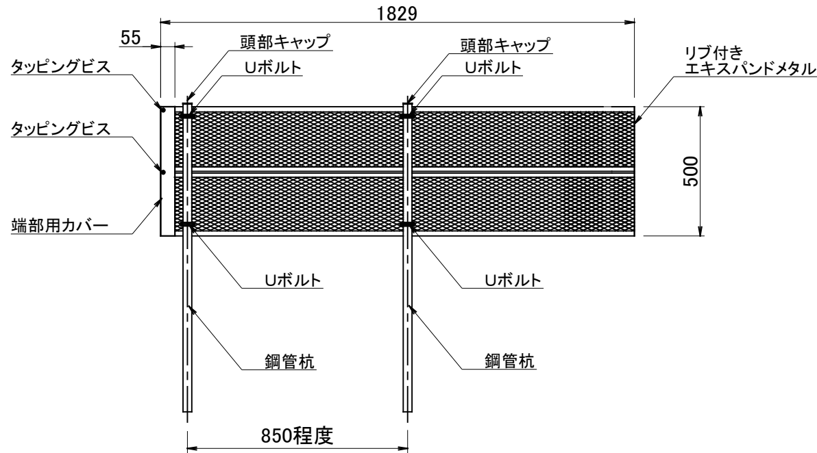
部品図
