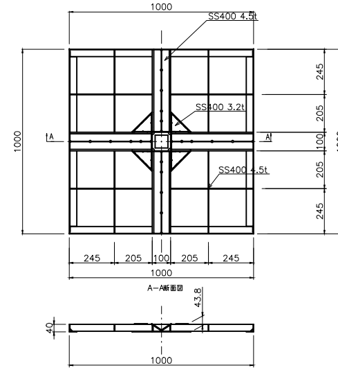
標準断面図 1:5
