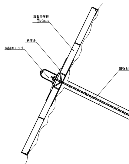
標準断面図 1:5
