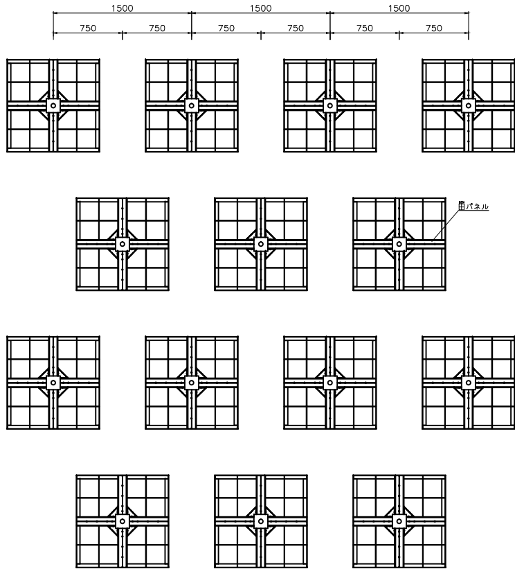
標準配置図 1:20
