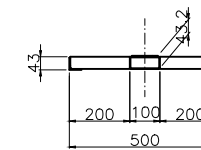
A-A断面図
