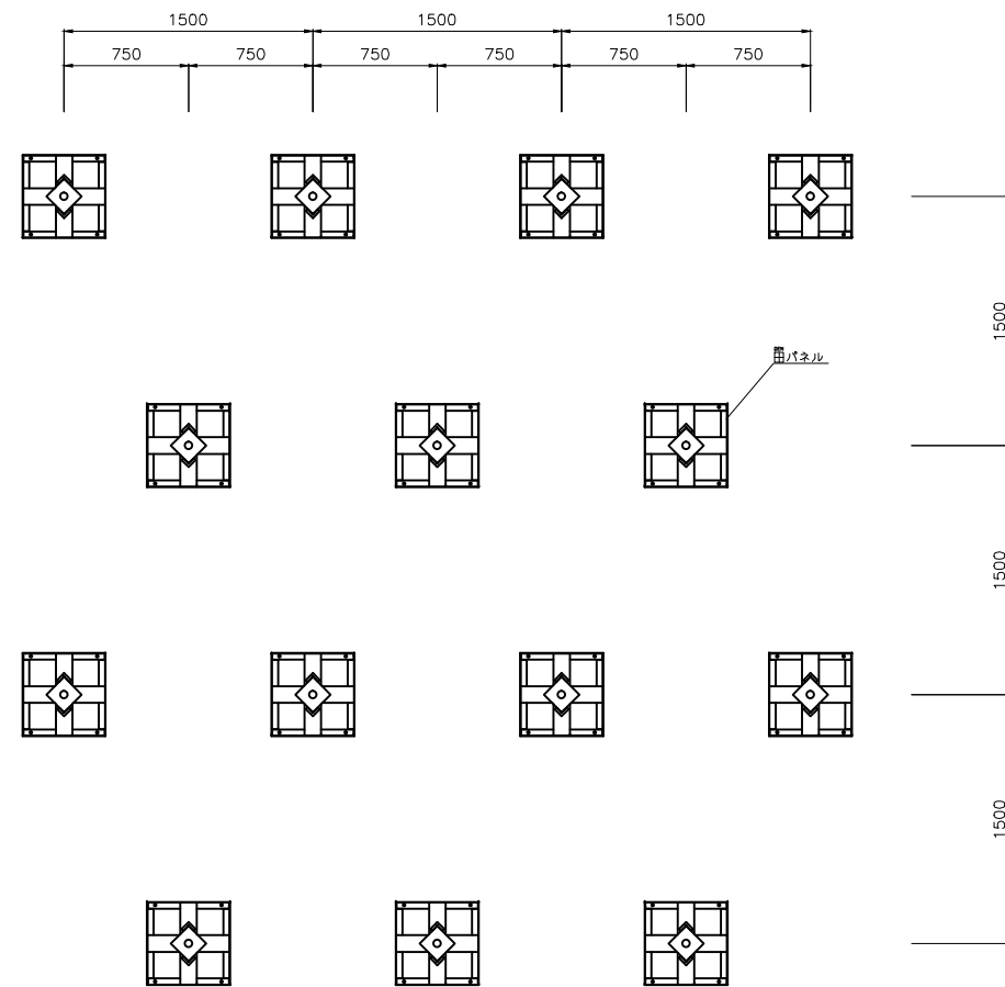
標準配置図 1:20
