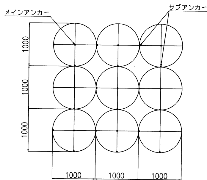
配置図 S=1/25
