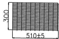
金網詳細図 S=1/2
