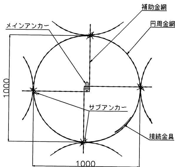
平面図 S=1/10
