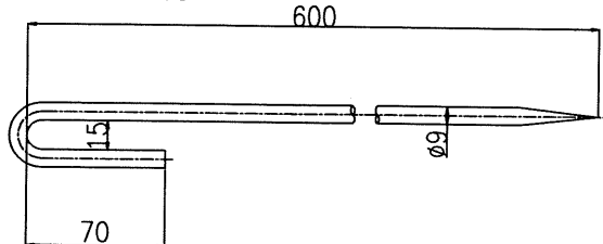
サブアンカー
