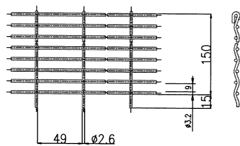
金網詳細図 S=1/2
