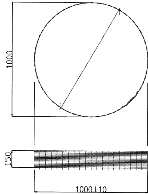
円周金網 S=1/10
