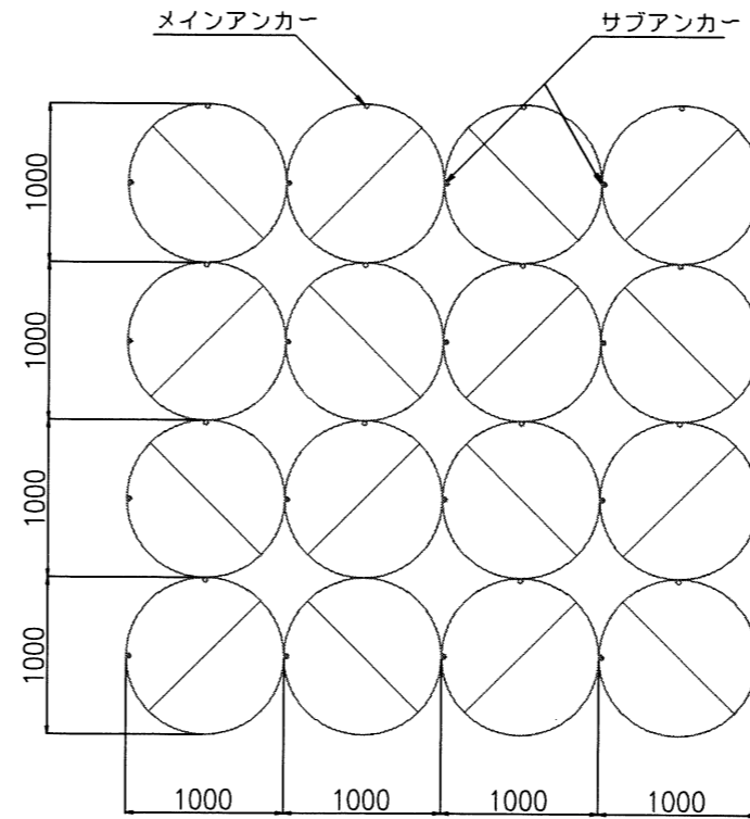
配置図 S=1/25
