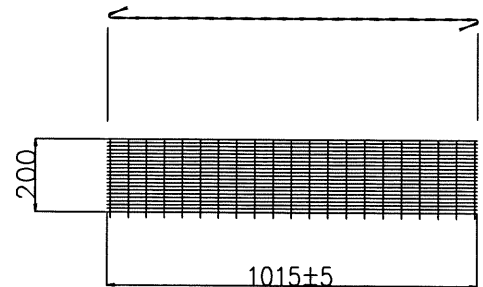
補助金網 S=1/10
