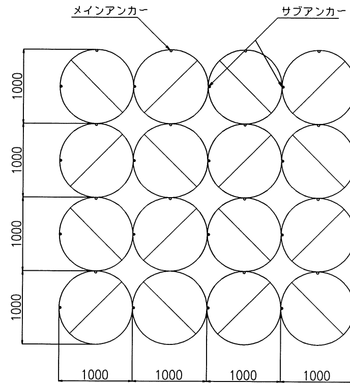
配置図 S=1/25
