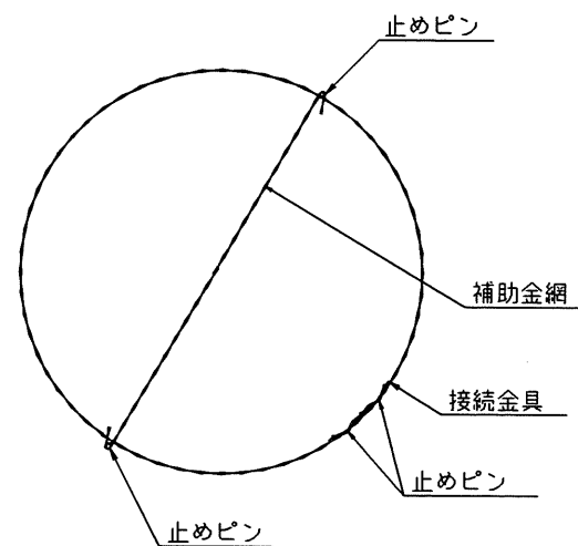
組立図 S=1/10
